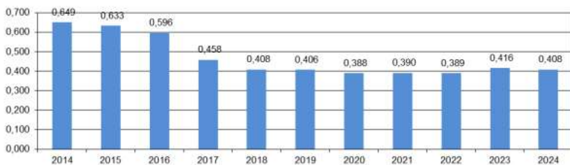
Потребление электроэнергии на 1 тонну товарной продукции, МВтч/тонна
