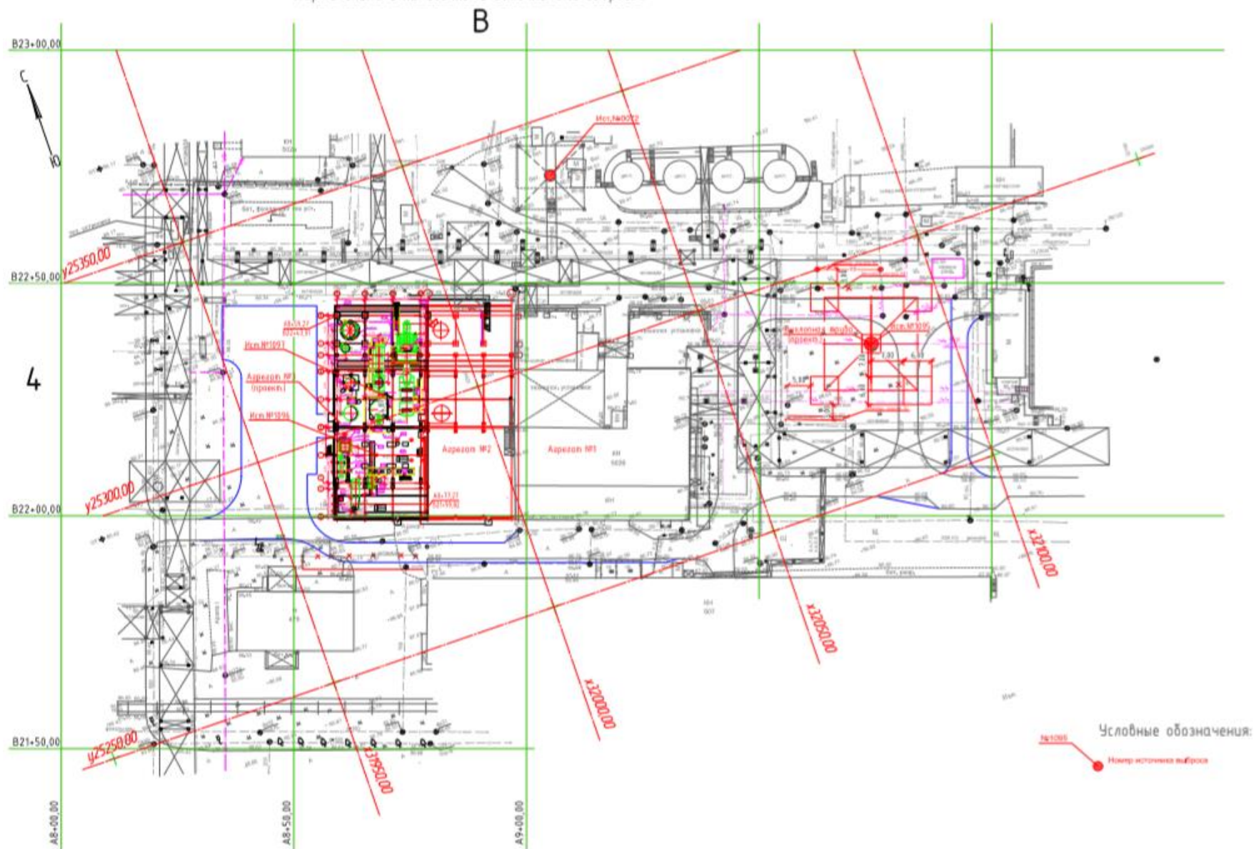
Рис. 3 Карта-схема промплощадки с нанесенными источниками выбросов
